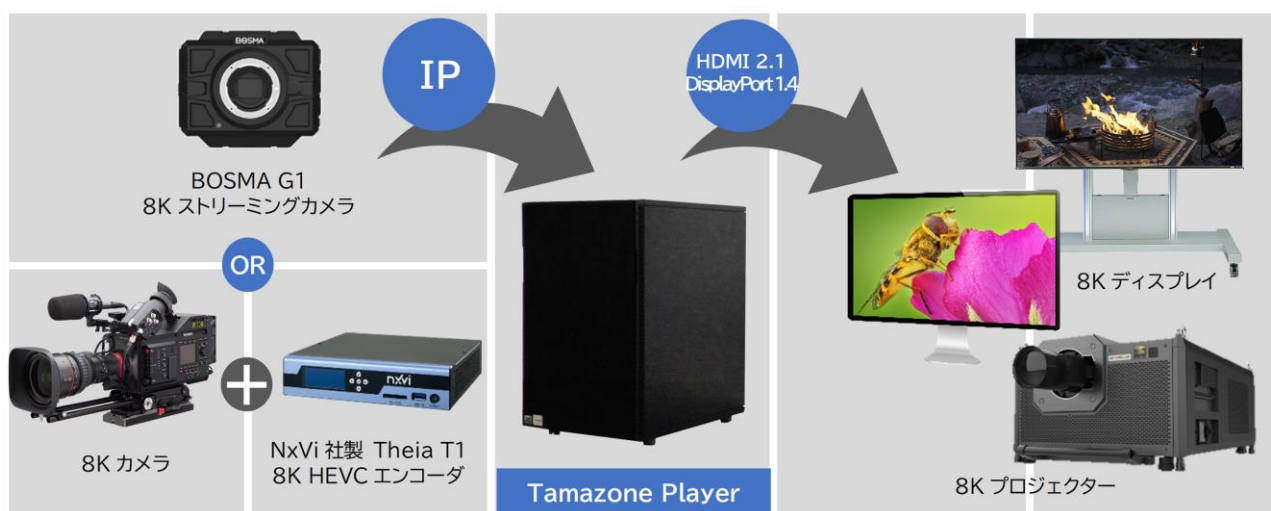
8K 伝送システム構成
